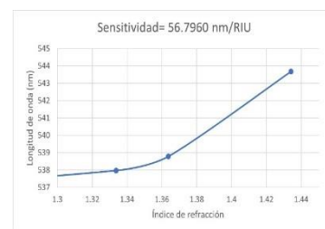
Figura 2. Sensibilidad del sensor 1 igual a 56.7960 nm/RIU.
