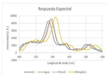
Figura 1. Respuesta espectral del sensor 1 operando a una longitud de onda de 535 nm y diámetro igual a 45 micrómetros.
